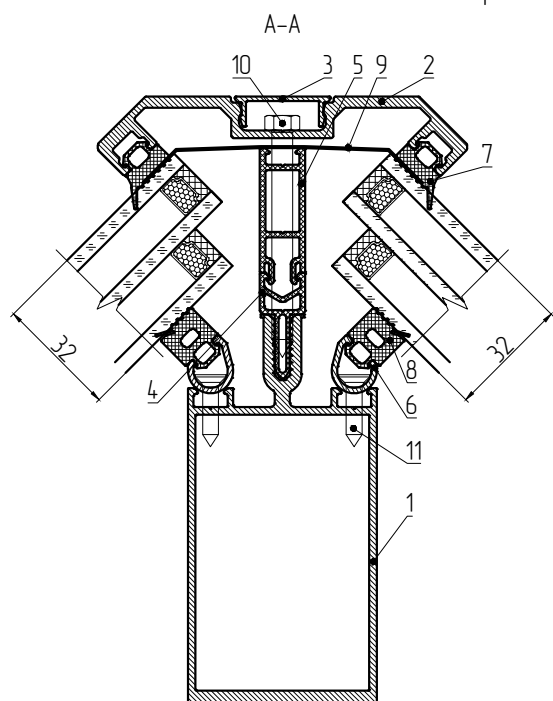
Угол поворота 90°. Вариант со стойкой МП-50311. Заполнение 24 мм
