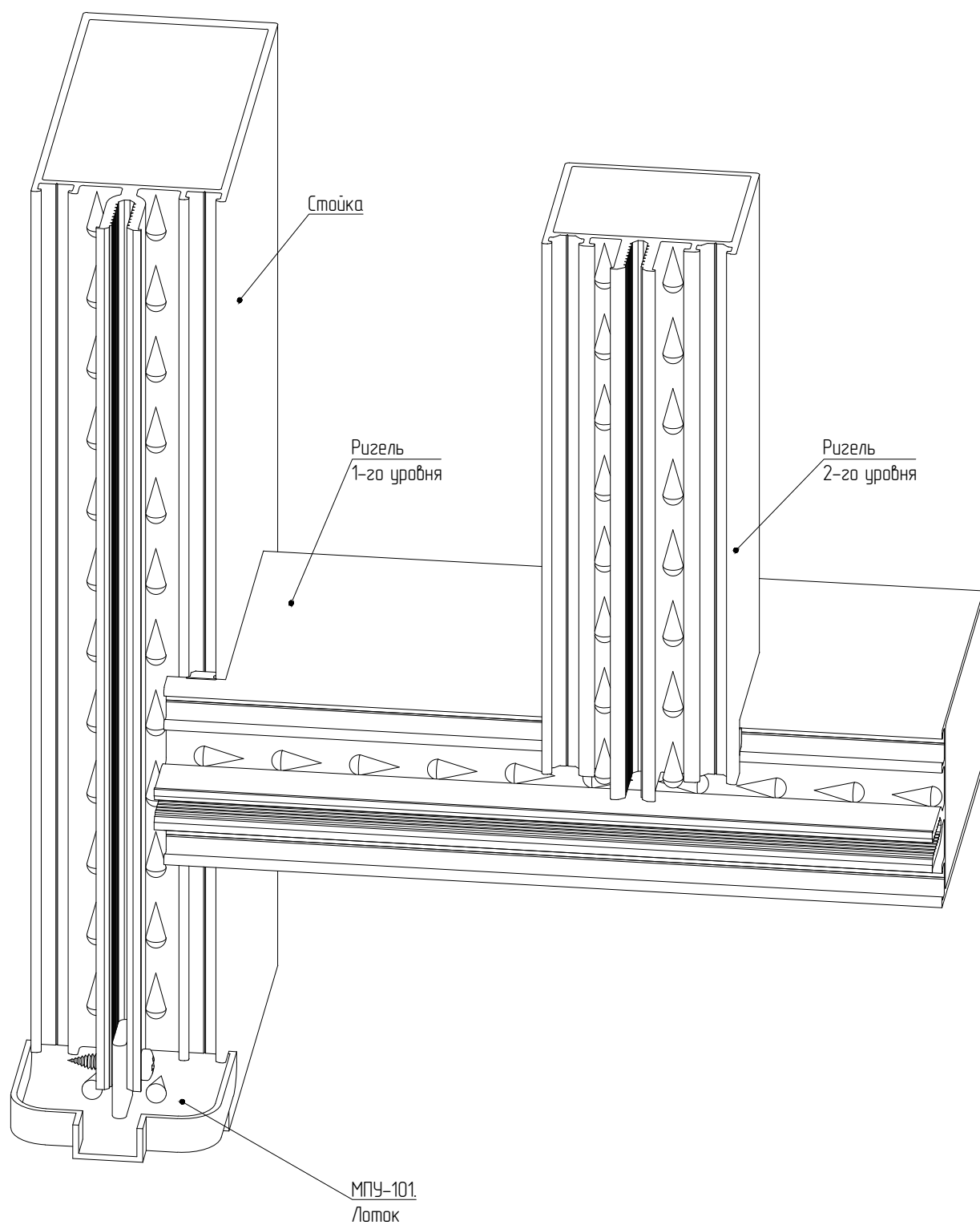
СХЕМА ОТВОДА ВЛАГИ Отвод влаги с лотка МПУ-101
