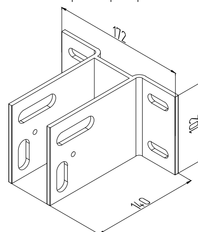
Габаритные размеры
